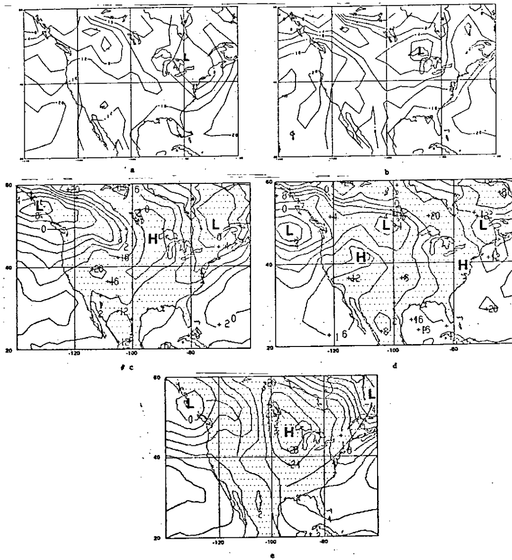
Fig. 16.2 - Campos de pressão ao nível do mar em 14 de Fevereiro de 1976, 0000 TMG.
