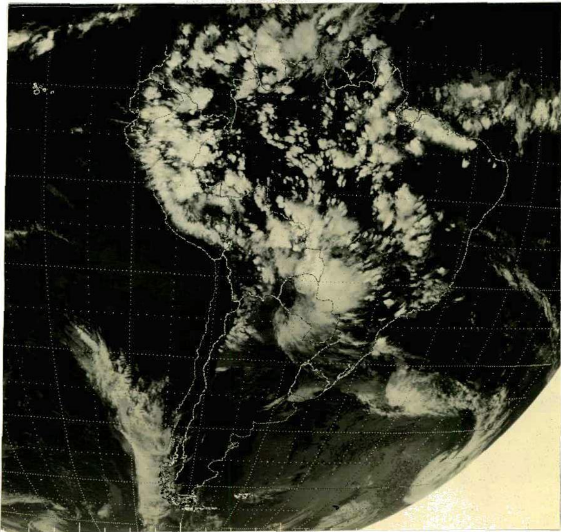
Fig. 17.17 - Linhas de instabilidade associadas à penetração da brisa marítima na Costa Norte do Brasil, imagem no infravermelho.
