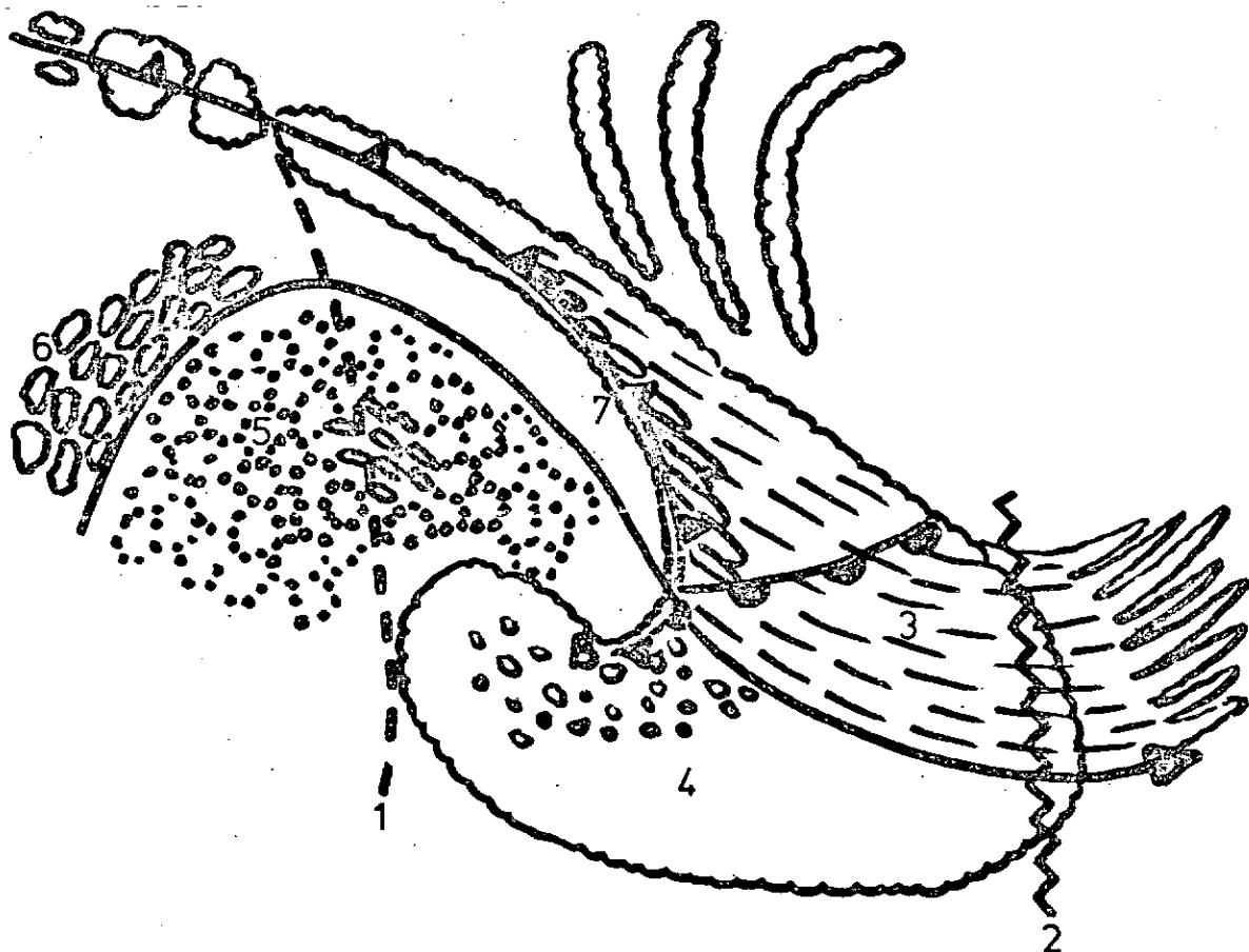
Fig. 17.19 - Configuração da nebulosidade associada a um sistema típico de latitudes médias.
