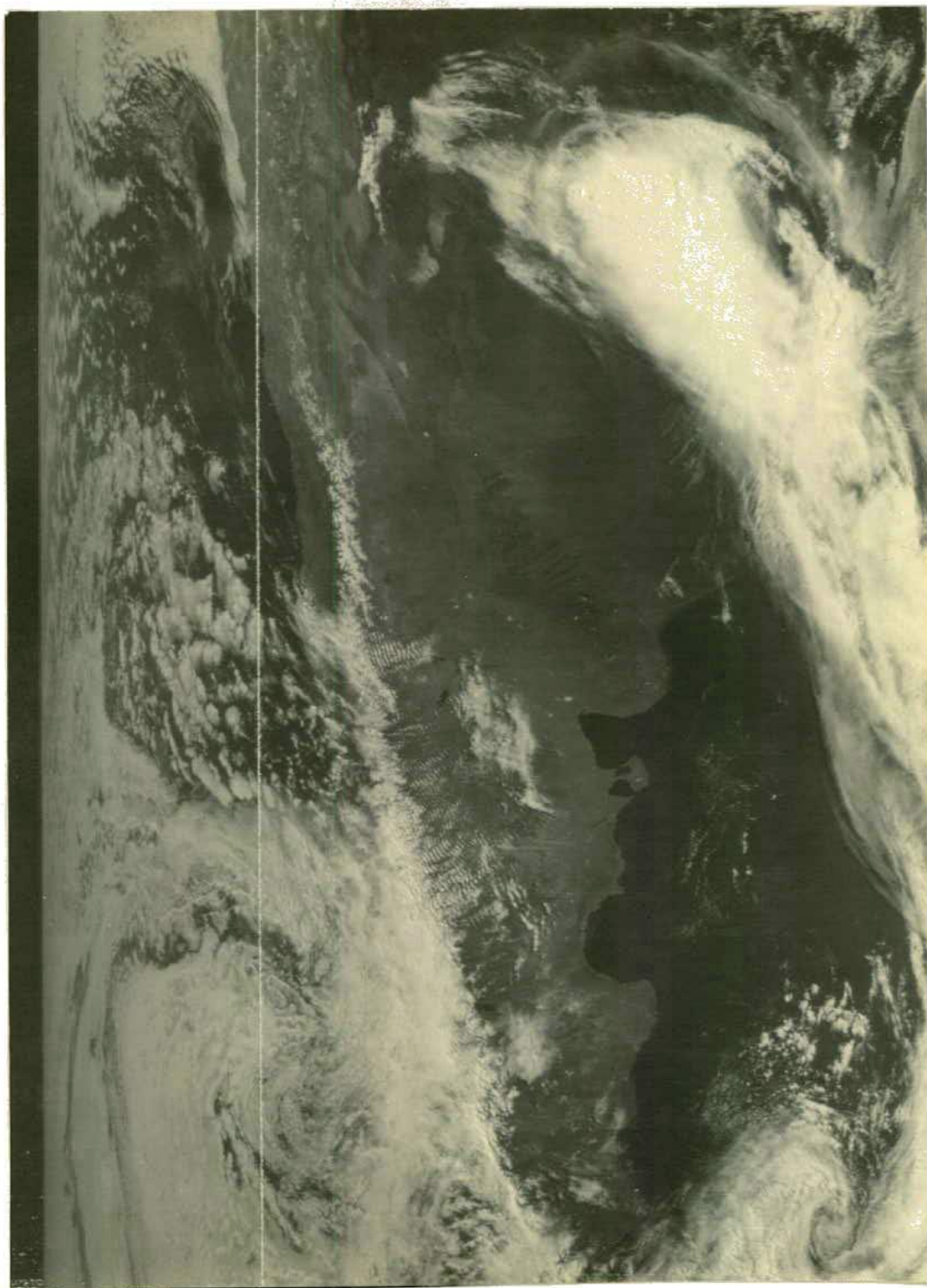
Fig. 17.15 - Nuvens altocumulus em forma de ondas a sotavento dos Andes, vistas numa imagem no visível.
