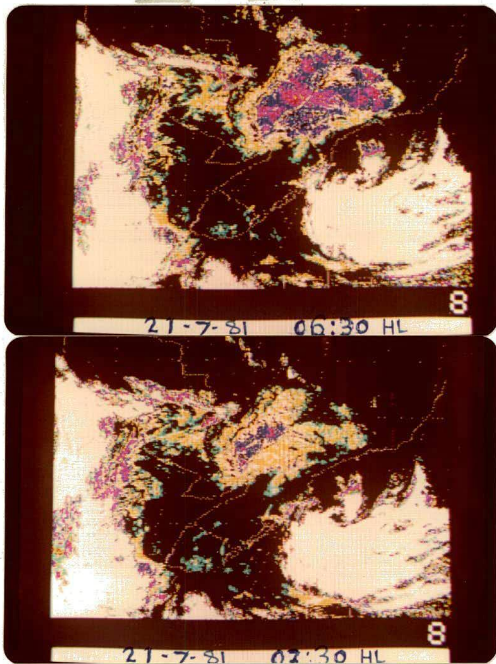
Fig. 15.5 - Imagens realçadas da temperatura da superfície terrestre durante a noite da geada severa no Brasil, 20 a 21 de julho de 1981, 6:30 e 7:30 HL.
