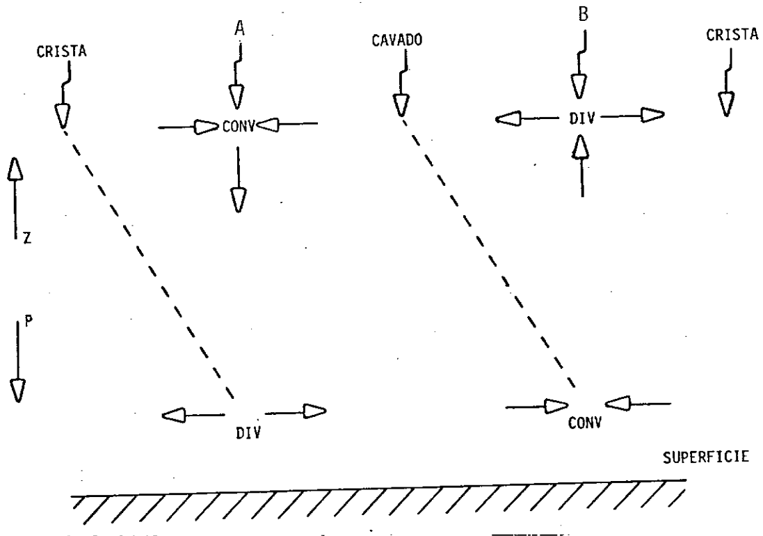
Fig. 17.5 - Corte este-oeste, tomado a partir do eixo da crista na Figura 17.4, passando pelos pontos A e B, até o eixo da próxima crista. (A inclinação vertical dos sistemas de pressão para oeste é ilustrada pelas linhas interrompidas).
