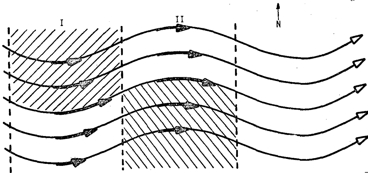
Fig. 17.3 - Configuração do escoamento na troposfera média ou superior, em função do cisalhamento e da curvatura horizontal.
