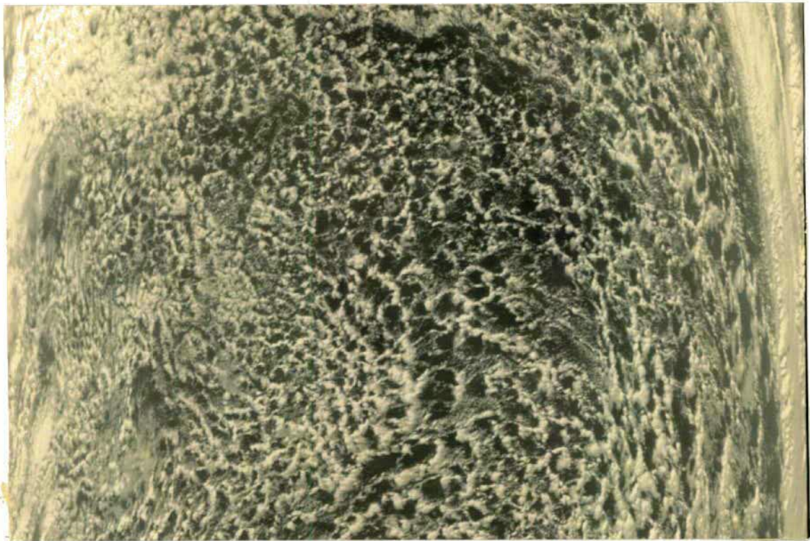
Fig. 17.8 - Imagem no visível, mostrando células abertas associadas ao forte aquecimento por baixo de uma massa de ar frio.
