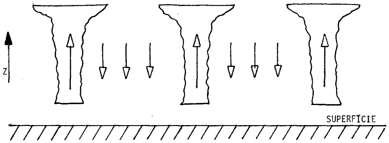
Fig. 17.7 - Movimento convectivo associado ao forte aquecimento por baixo.
