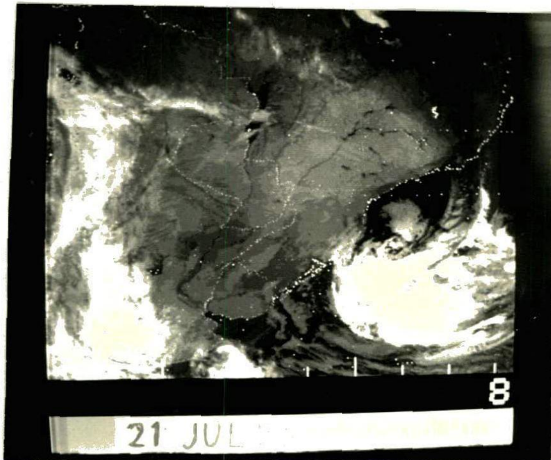
Fig. 15.2 - Imagem convencional do satélite SMS, no infravermelho, região Sul do Brasil às 6:00 HL do dia 21 de julho de 1981. - Um mapa é superposto. Esta imagem foi fotografada da tela de TV em preto e branco do UAI.
