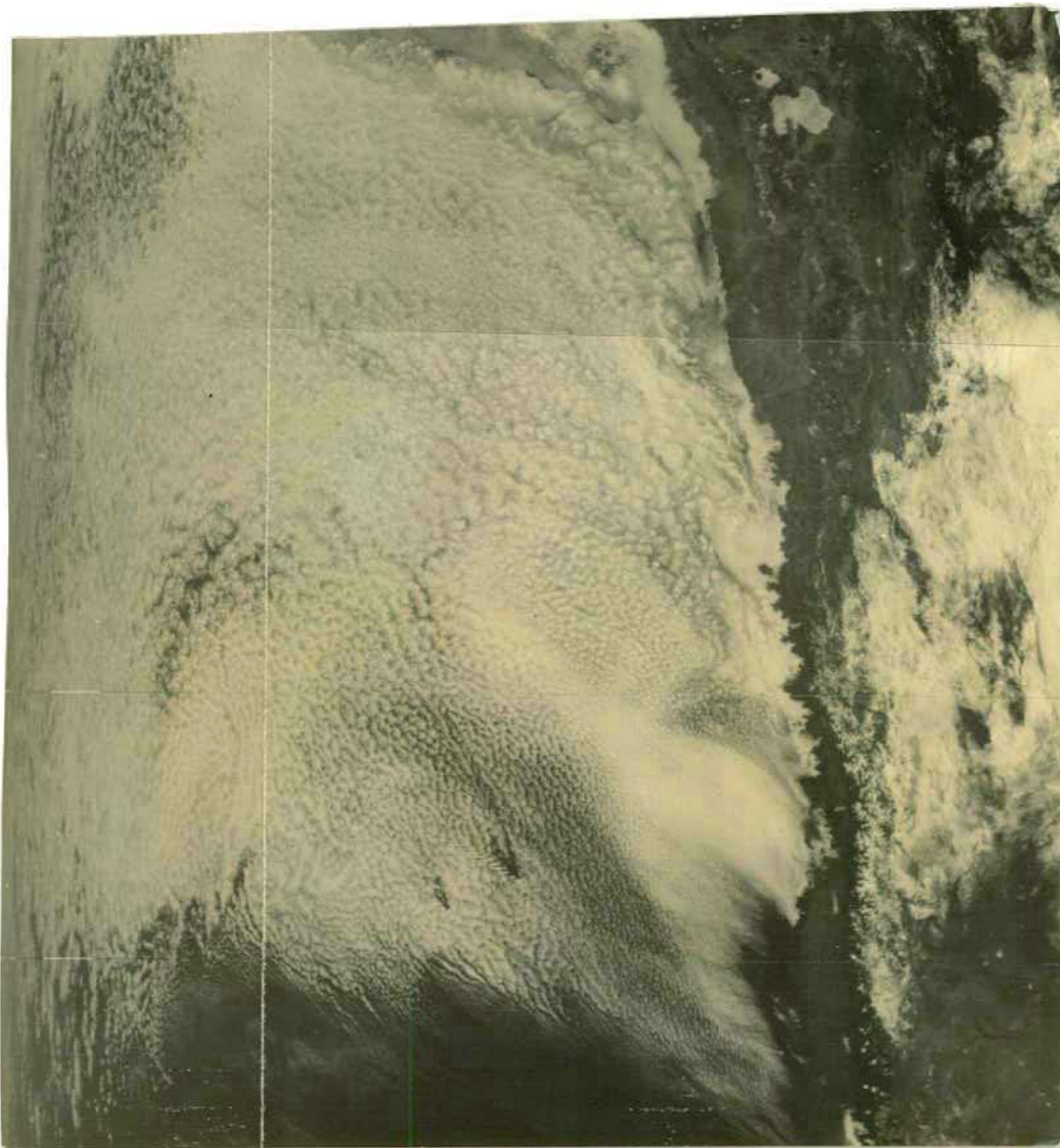
Fig. 17.10 - Imagem no espectro visível, mostrando células fechadas no Oceano Pacífico.
