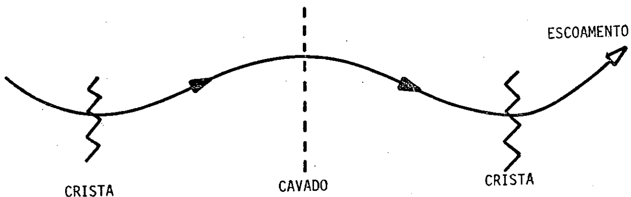
Fig. 17.1 - Configuração típica do escoamento ondulatório da troposfera média e superior, para o Hemisfério Sul.
