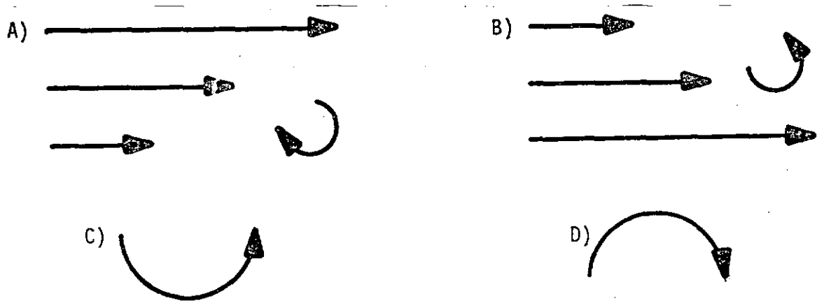
Fig. 17.2 - Diagramas esquemáticos da vorticidade, para o Hemisfério Sul, de (A) vorticidade devida ao cisalhamento ciclônico; (B) vorticidade devida ao cisalhamento anticiclônico; (C) vorticidade devida à curvatura anticiclônica; (D) vorticidade devida à curvatura ciclônica.
